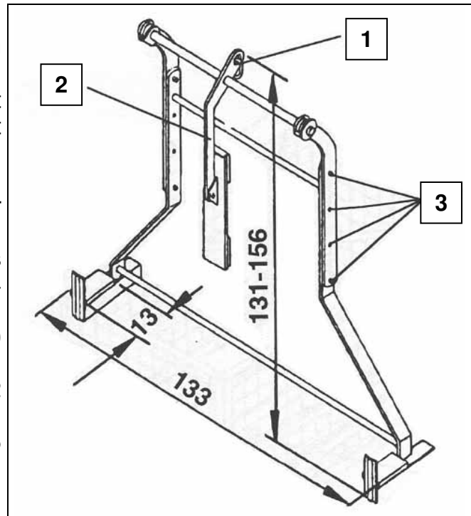
Fig. 23 Plattengreifer
