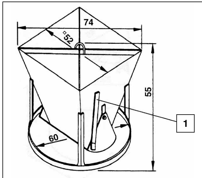
Fig. 19 Mörtelsilo 65 Liter
