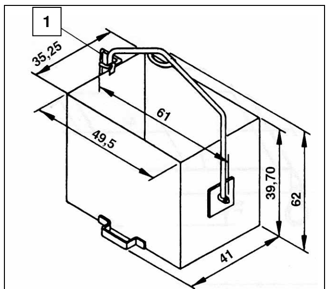
Fig. 18 Kippkübel 65 Liter
