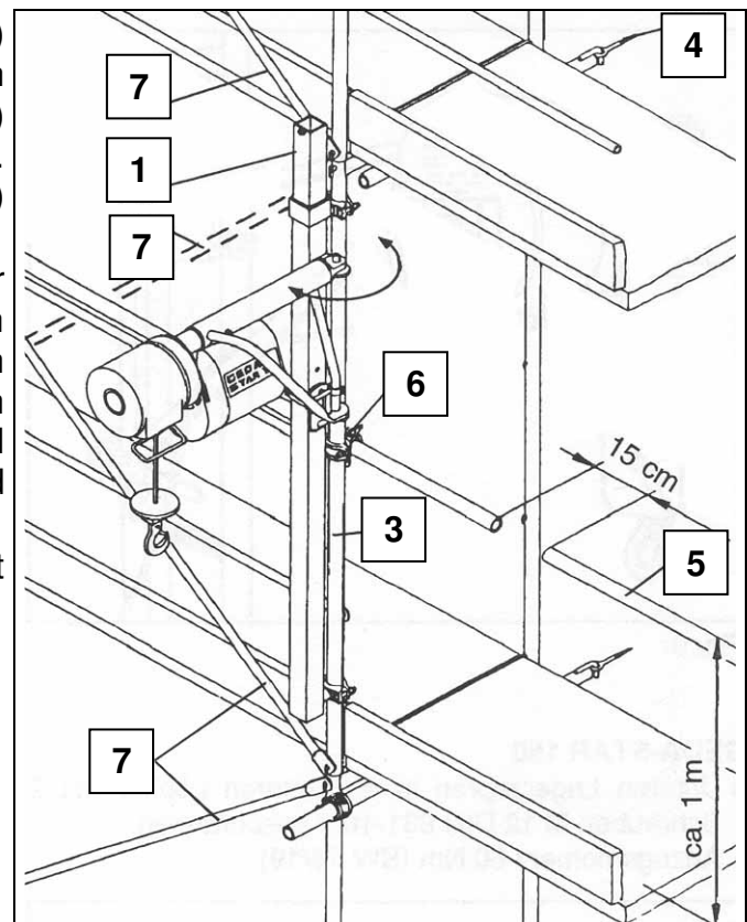
Fig. 11 Gerüstbefestigung montieren
