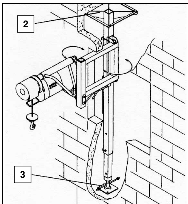
Fig. 13 Geschossstütze montieren
