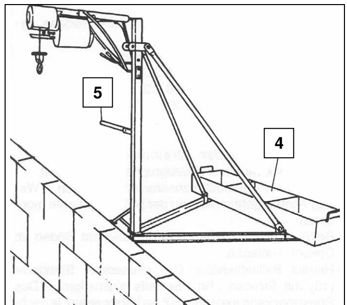
Fig. 9 Dreibock positionieren
