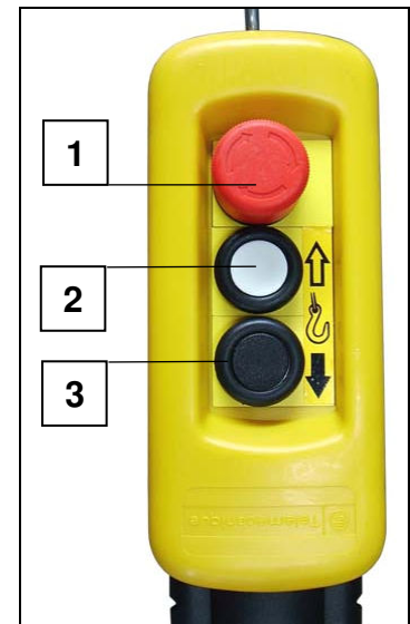
Fig. 24 Bedienung/Steuerung
